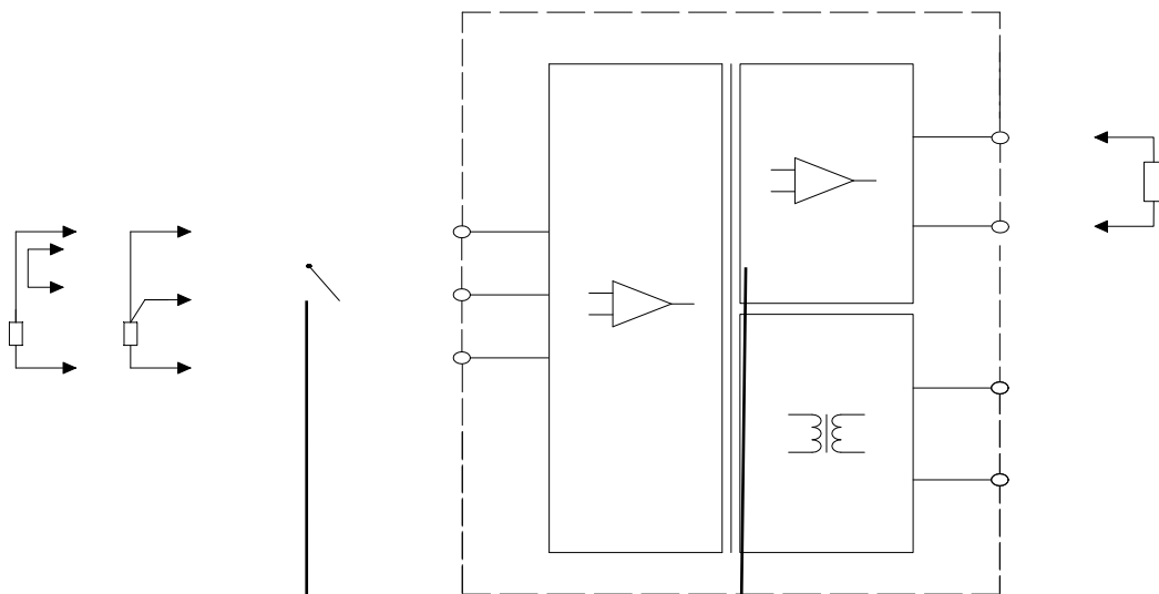
单入单出接线图
